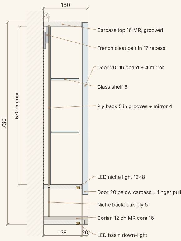
SECTION A-A · SW-MC-100
